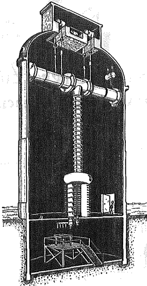
Gleichrichteranlage für 1200.kV Gleichspannung mit darüberlie- gendem Transformator (Entwurf)
